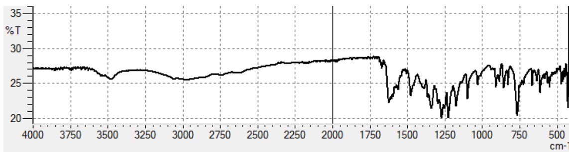
Hình 8 Phổ IR của hợp chất A1
