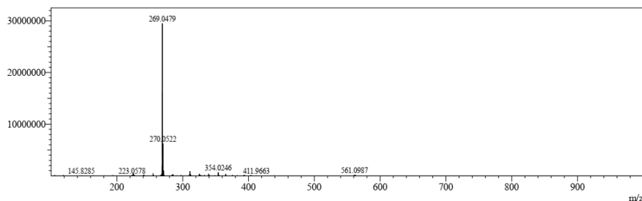
Hình 9 Phổ MS (ES + ) của hợp chất A1
