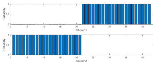
Hình 8. Xác suất thuộc vào hai cụm của 42 phần tử
